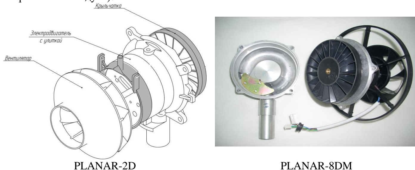
Рис.11 – Нагнетатель воздуха
