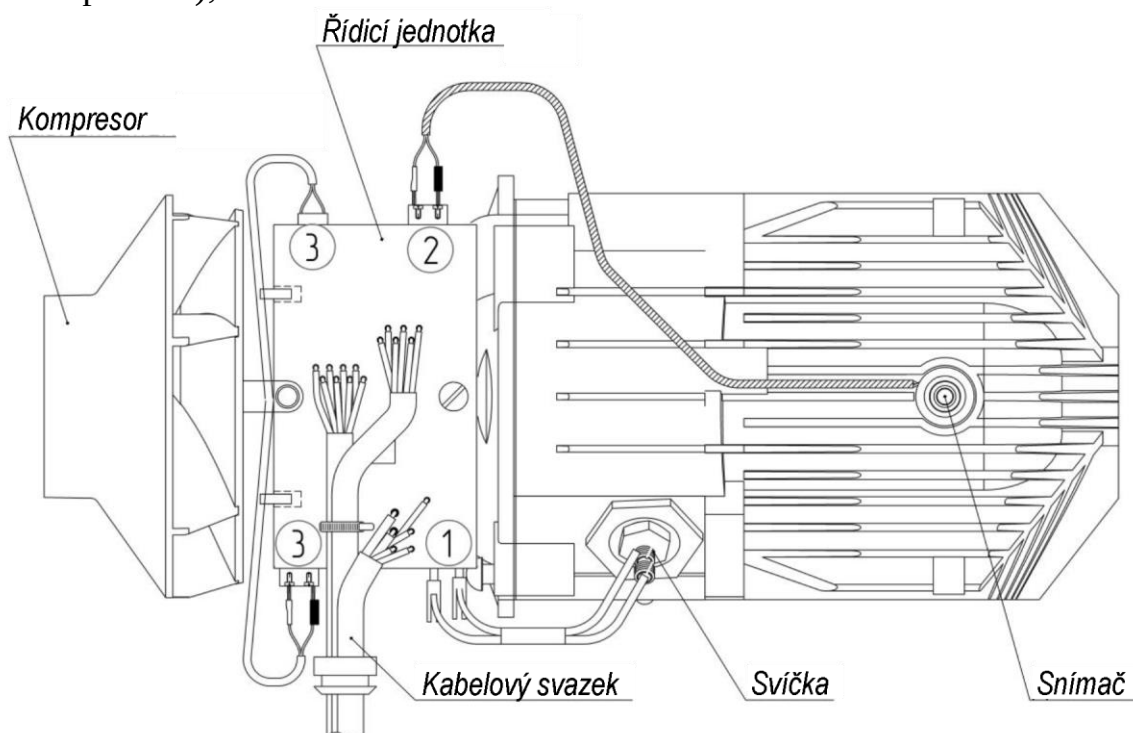
Obr. 2 - Ohřívač.
