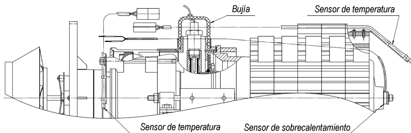
Fig.10 – Sensori.
