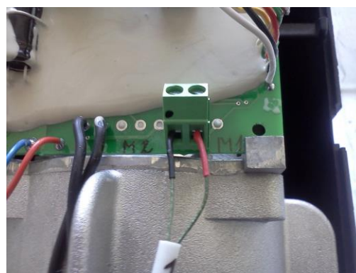
Fig. 9a – Connessione
