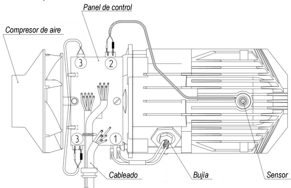
- Fig.2 – Riscaldatore.
