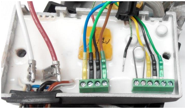
Rys.6a – Zworka
