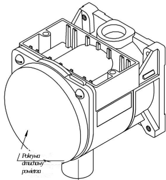
Rys. 7 - Dmuchawa powietrza
