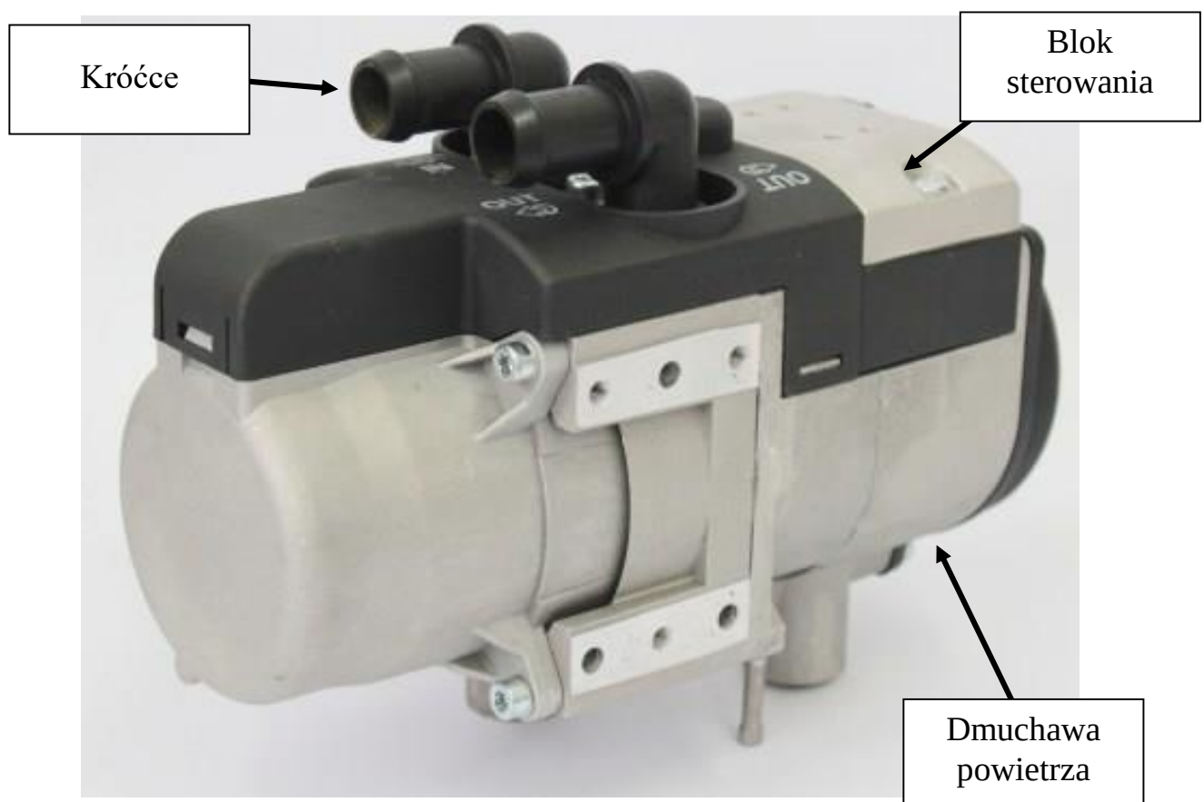
Rys.1 – Nagrzewnica
