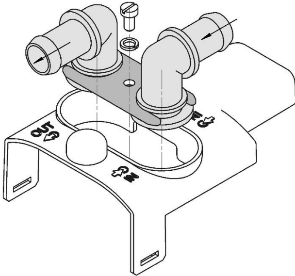
Rys.2 – Demontaż zacisku
