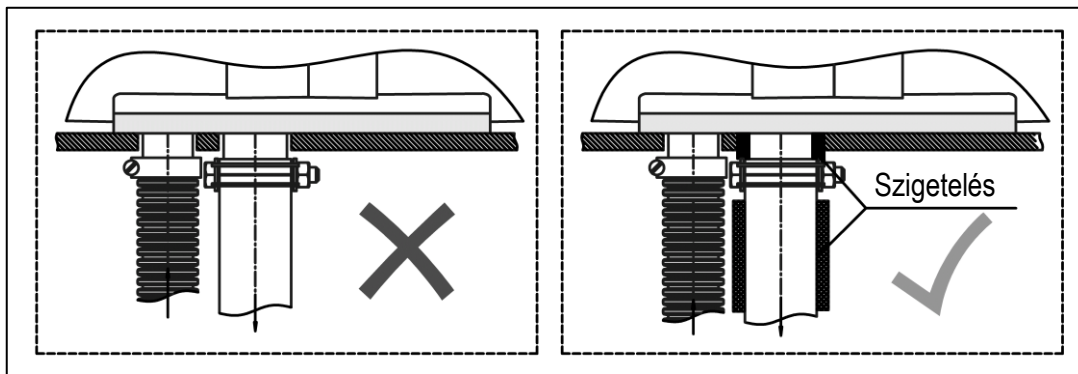
12. ábra - Kiegészítő hőszigetelés beszerelése
