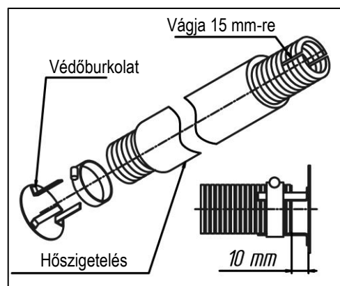
9. ábra - A kipufogócső védőburkolata
