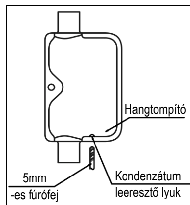
10b ábra - Kondenzátum leeresztő nyílása függőleges beszereléshez
