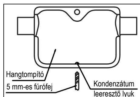
10a ábra - Kondenzátum leeresztő nyílás vízszintes beszereléshez
