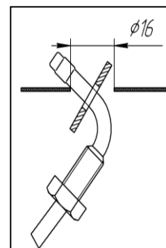
Obr. 15b – Instalace podložky
