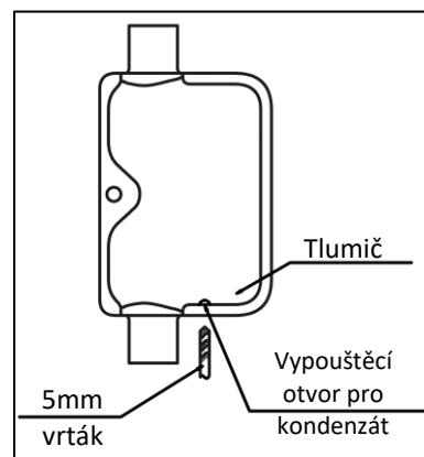
Obr. 10b – Vypouštěcí otvor kondenzátu pro vertikální montáž
