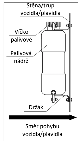
Obr. 16 – Instalace palivové nádrže
