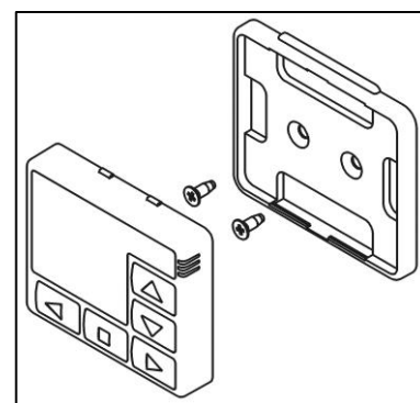
Obr. 24 – Instalace ovládacího panelu PU-27 s použitím montážního držáku
