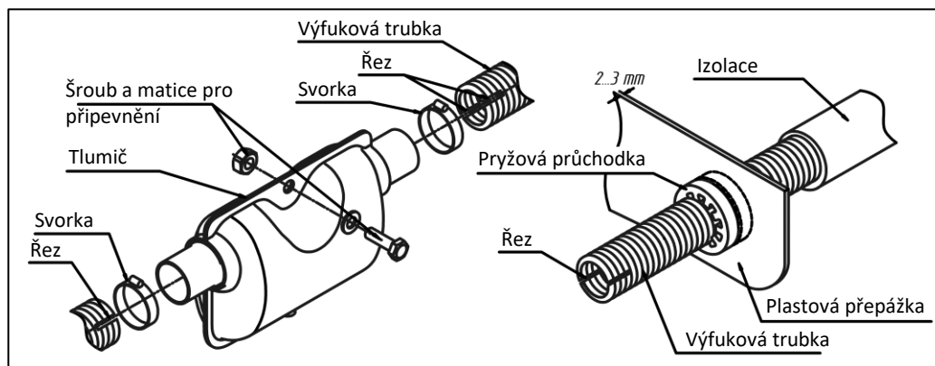
Obr. 11 – Připojení výfukového potrubí k ohřívači a použití pryžové průchodky
