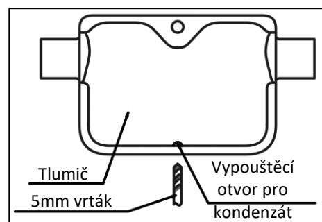
Obr. 10a – Vypouštěcí otvor kondenzátu pro horizontální montáž
