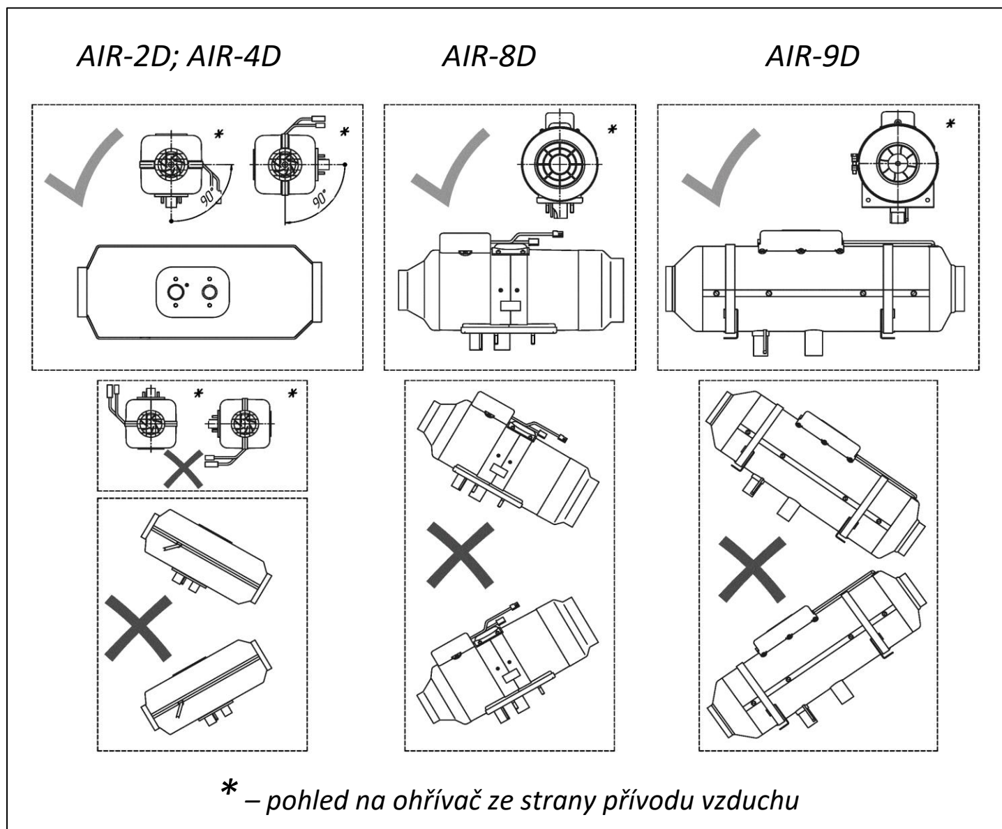
Obr. 1a – Montážní poloha ohřívače
