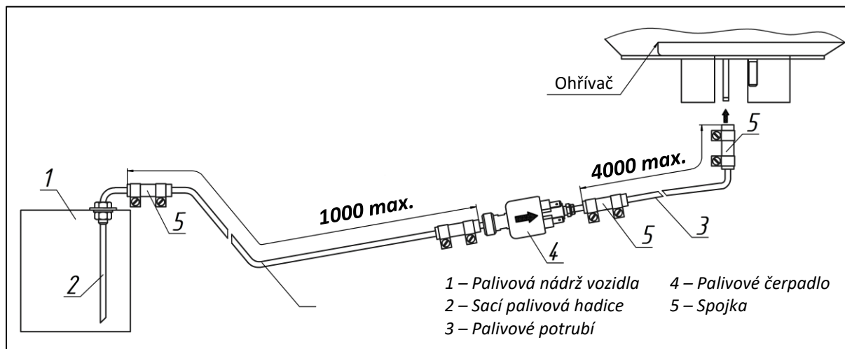
Obr. 14 – Příklad přívodu paliva do ohřívače pomocí sací palivové hadice
