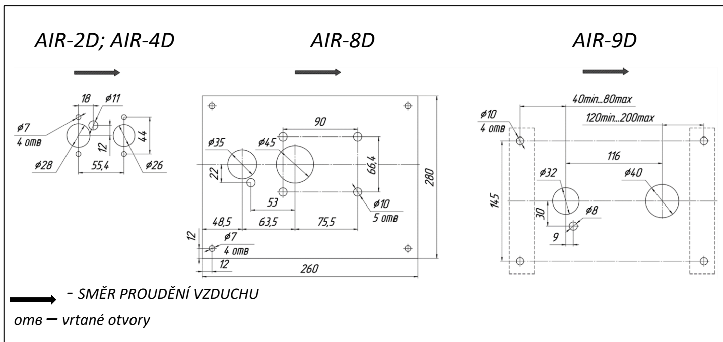
Obr. 3 – Montážní otvory
