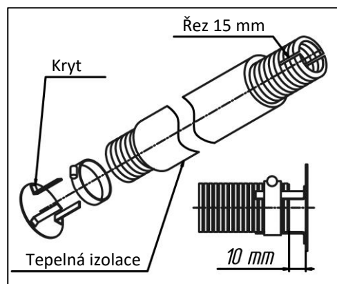
Obr. 9 – Kryt výfukového potrubí
