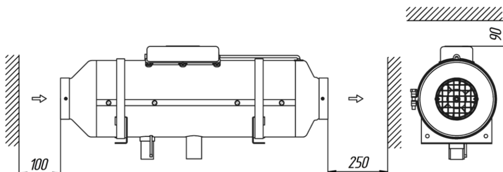
Obr. 1b – Vzdušenost od stěn
