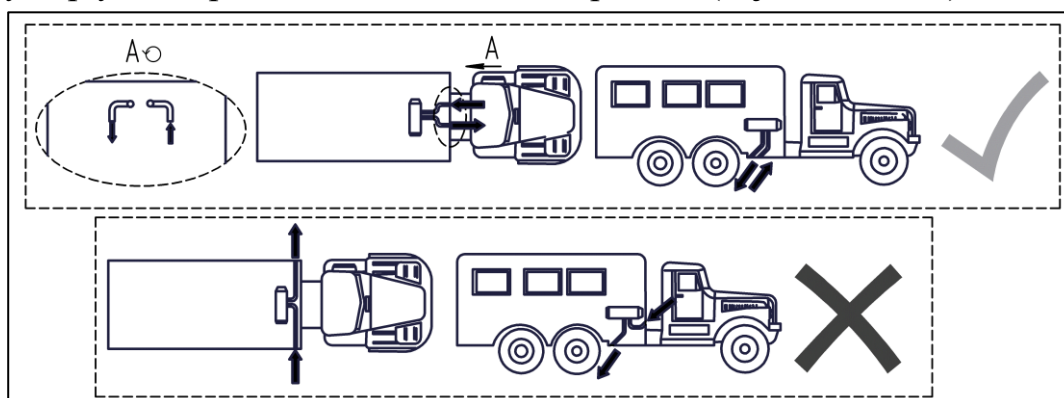
Obr. 6a – Umístění výfukového a přívodního vzduchového potrubí na pozemních vozidlech
