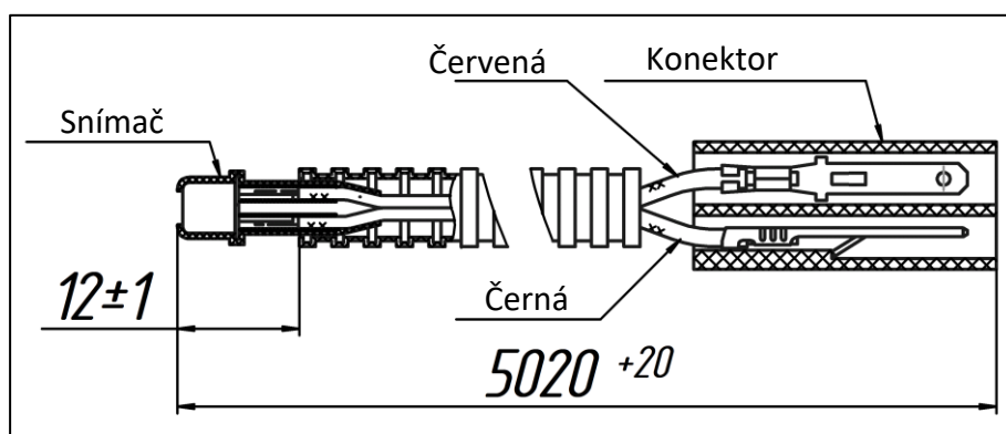
Obr. 23 – Teplotní snímač
