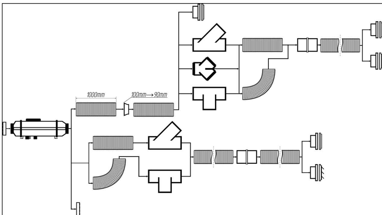
Obr. 26c – Připojení vzduchových potrubí pro AIR-9D (100/90 mm)
