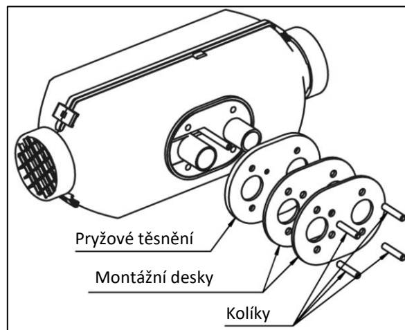
Obr. 2a – Montážní desky
