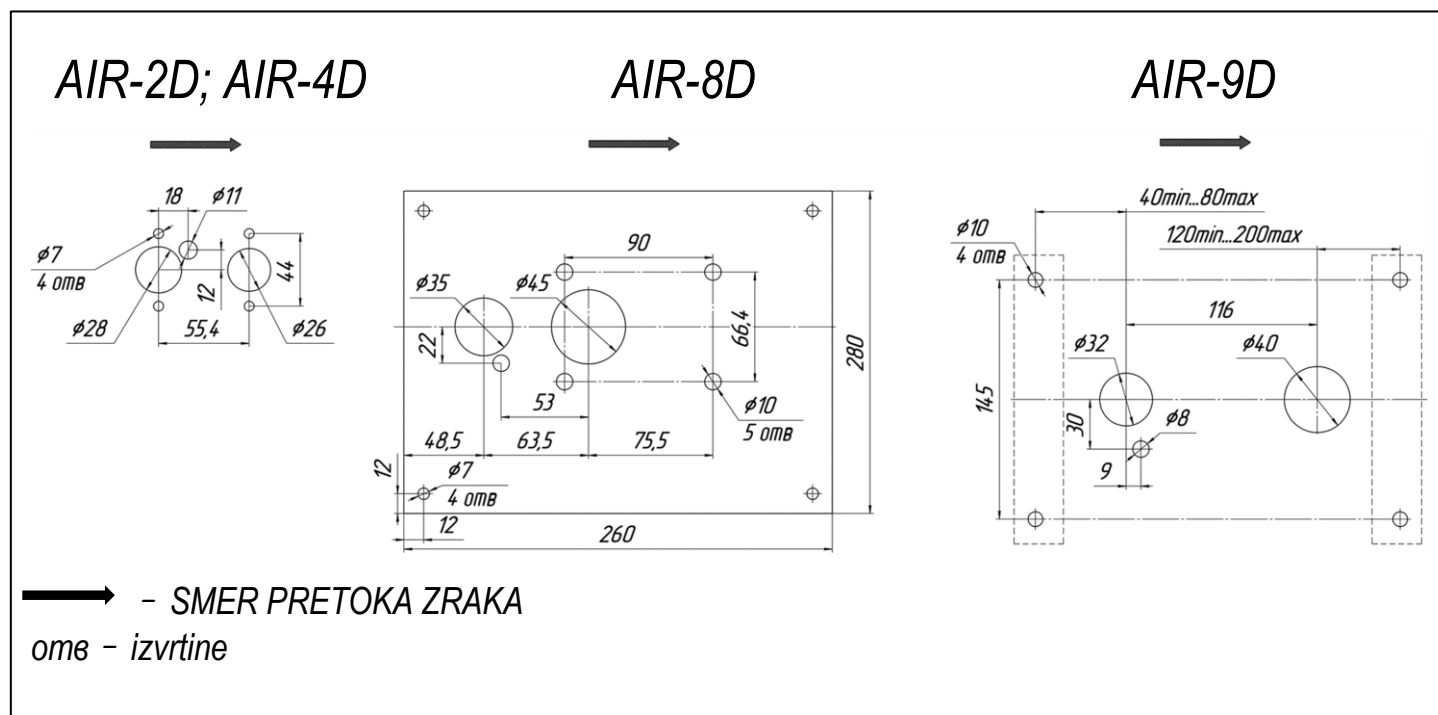
Slika 3 - Montažne luknje
