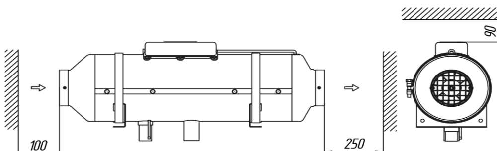
Slika 1b – Oddaljenost od sten
