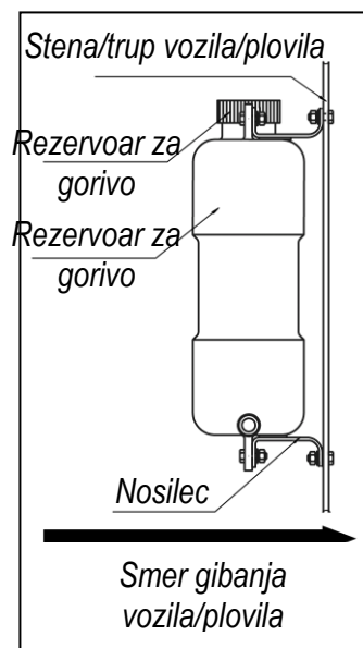
Slika 16 Namestitev rezervoarja za gorivo
