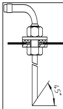
Slika 15a – Namestitev sesalne cevi za gorivo
