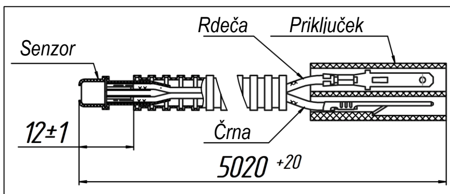
Slika 23 – Temperaturni senzor
