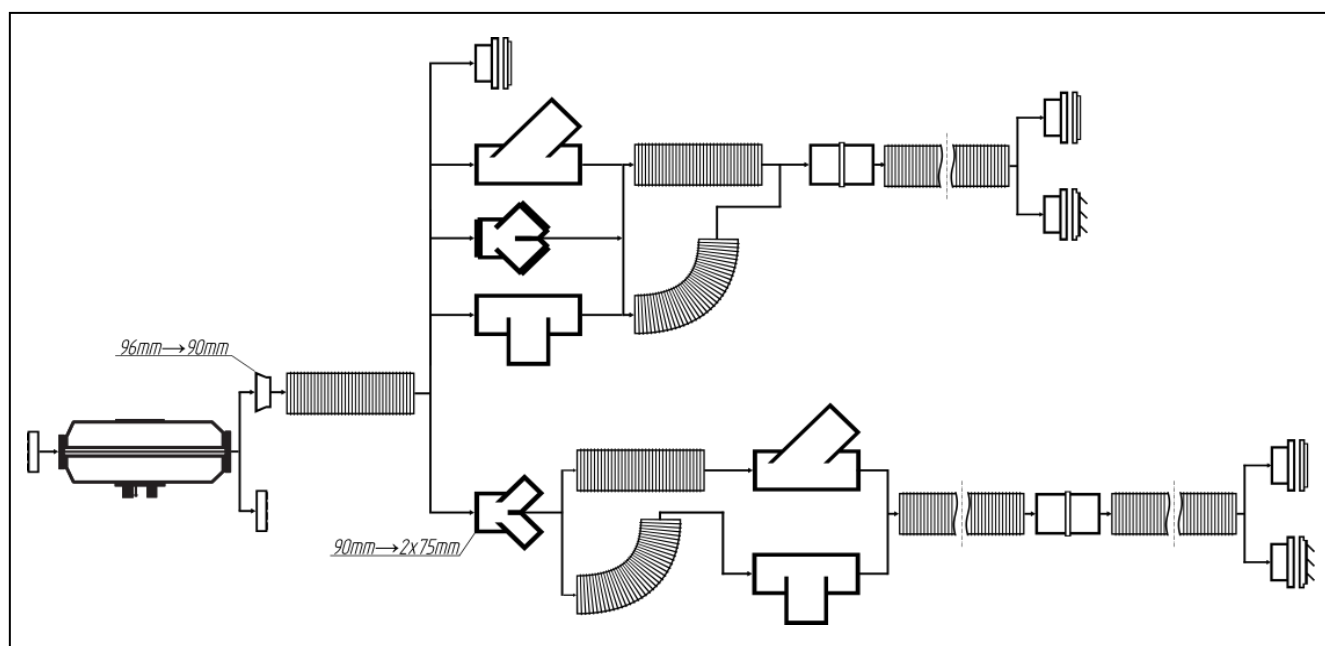
Рис. 26б – Соединения воздушного канала для AIR-4D (90 мм / 75 мм)
