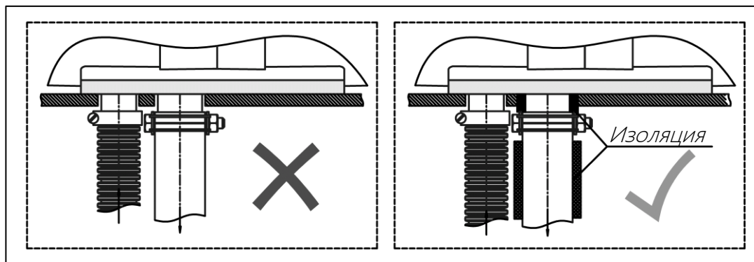
Рис. 12 – Установка дополнительной теплоизоляции
