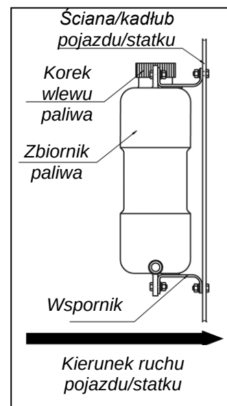
Rys. 16. Instalacja zbiornika paliwa.
