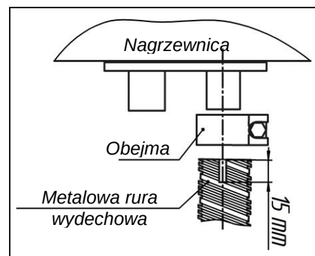
Rys. 8. Mocowanie metalowej rury do nagrzewnicy.
