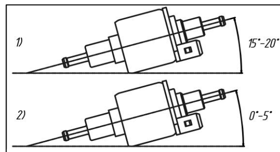
Rys. 18. Kąt montażu pompy paliwa Advers (1) i pompy paliwa Thomas Magnete (2).
