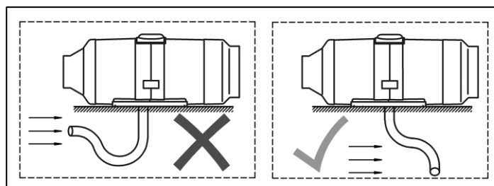
Rys. 5. Położenie rury wlotowej/wylotowej powietrza
