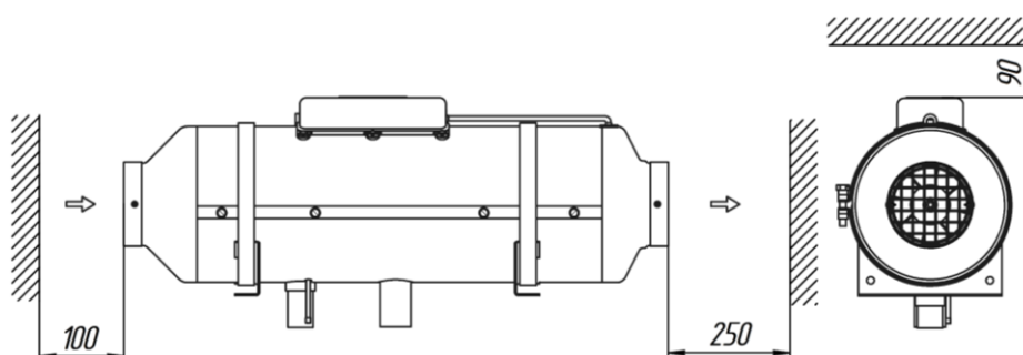
Rys. 1b. Odległość od ścian
