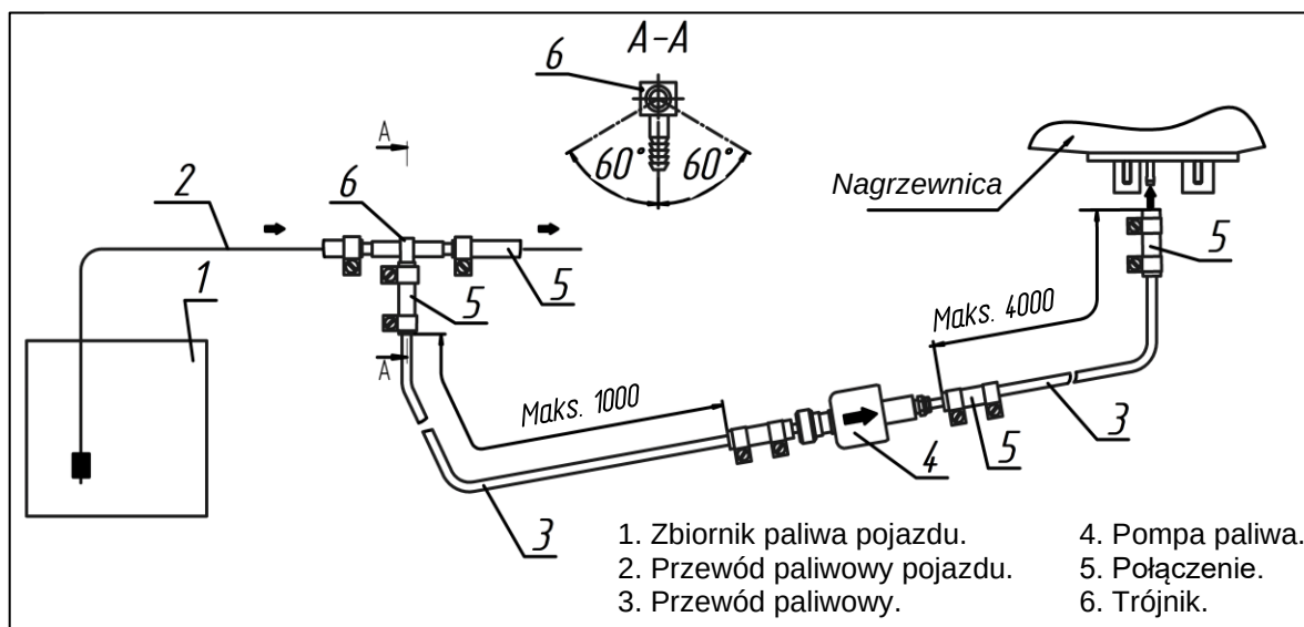
Rys. 17. Zasysanie paliwa za pomocą trójnika.
