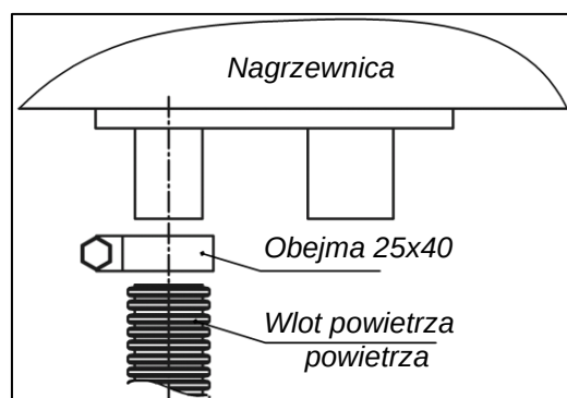
Rys. 4. Podłączenie rury powietrza do nagrzewnicy
