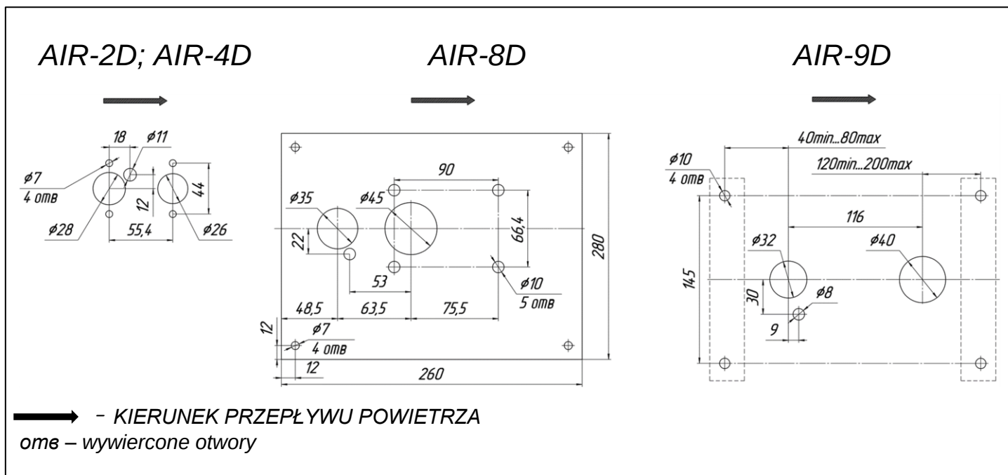
Rys. 3. Otwory montażowe
