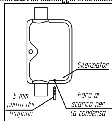
Fig. 10b - Foro di scarico per la condensa con montaggio verticale
