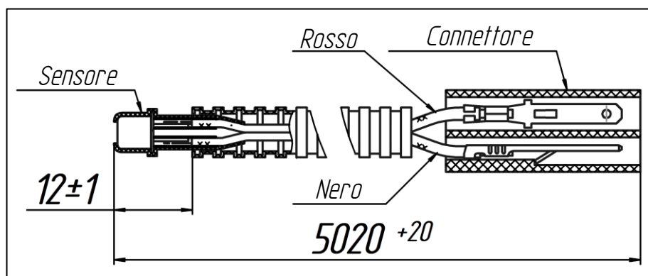
Fig. 23 - Sensore della temperatura
