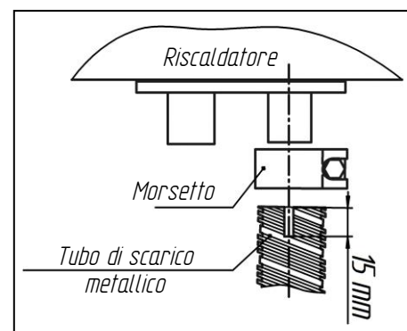
Fig. 8 - Collegamento del tubo metallico al riscaldatore
