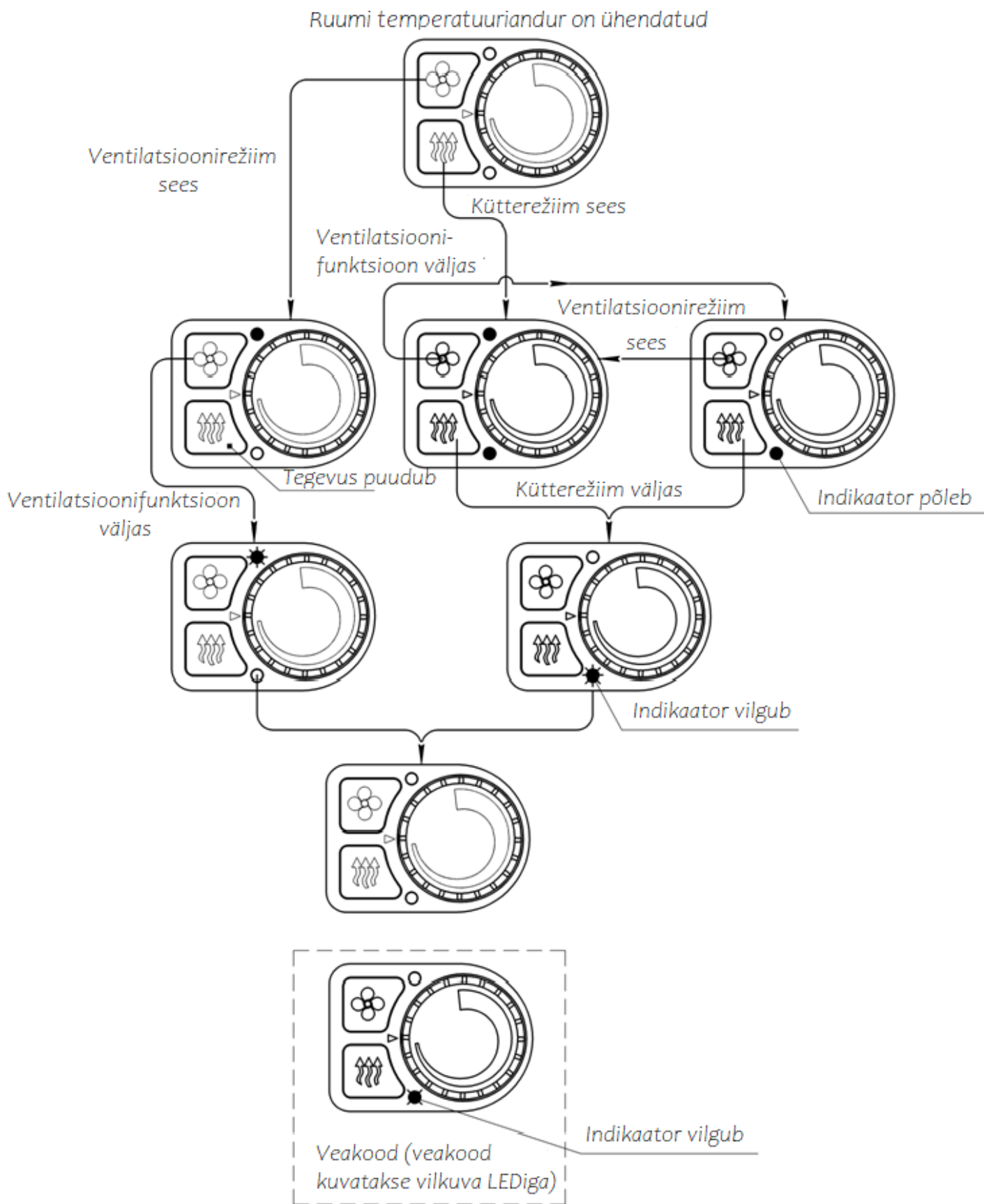
Kontrolloperatsiooni diagramm
